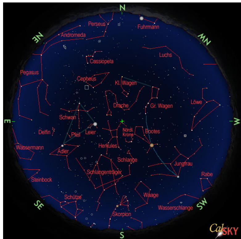
Sommerlicher Sternhimmel für Deutschland: Ende Juni 23h MESZ, bzw. Ende Juli 21h MESZ
